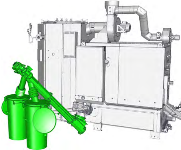
Fig. 7-4: Décendrage dans 2 fûts à cendres
