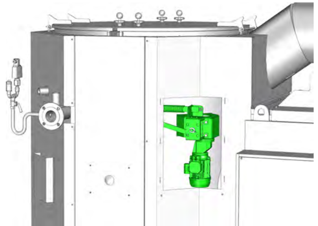
Fig. 7-1: Entraînement du dispositif de nettoyage de l'échangeur de chaleur
