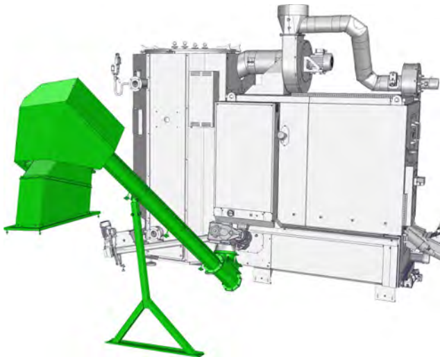
Fig. 7-5: Décendrage à l'aide d'un clapet de transfert
