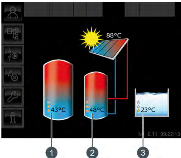
Fig. 8-24: Installation solaire avec 3 accumulateurs
