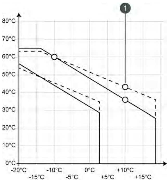
Fig. 8-18: Adapter la courbe de chauffage au cours de la période de transition
