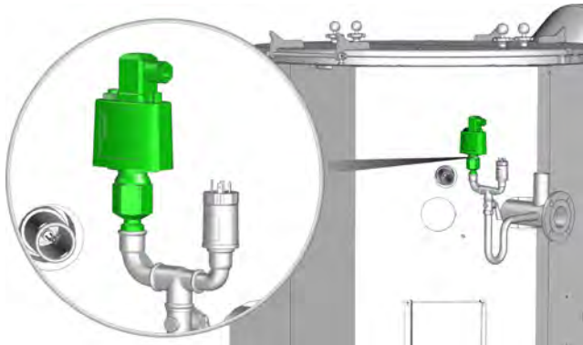
Fig. 6-3: Limiteur de pression minimale
