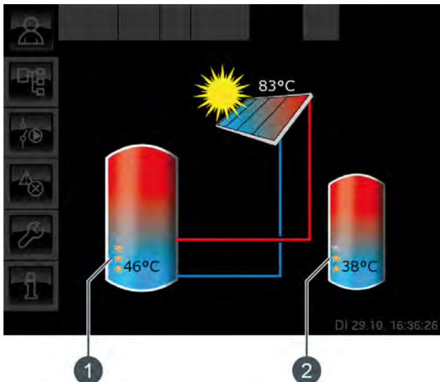
Fig. 8-23: Installation solaire avec 2 accumulateurs
