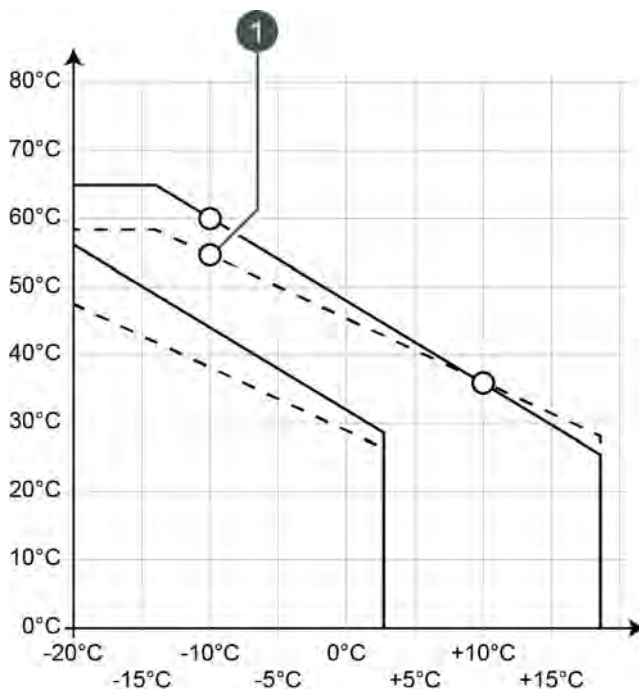
Fig. 8-19: Adapter la courbe de chauffage en hiver
