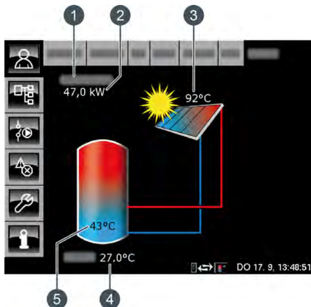
Fig. 8-22: Installation solaire avec un accumulateur
