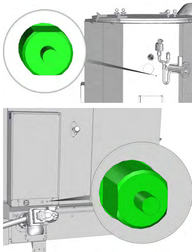
Fig. 6-1: Positions de déverrouillage des deux limiteurs de température de sécurité
