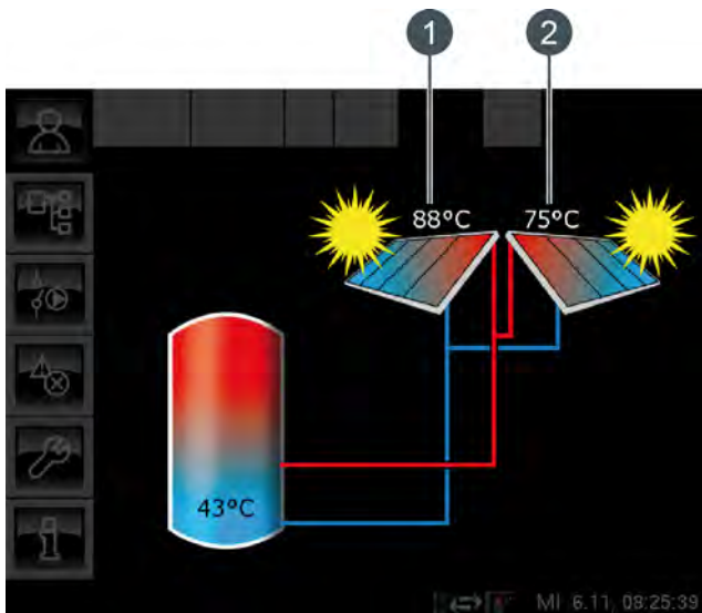
Fig. 8-28: Installation solaire avec deux collecteurs
