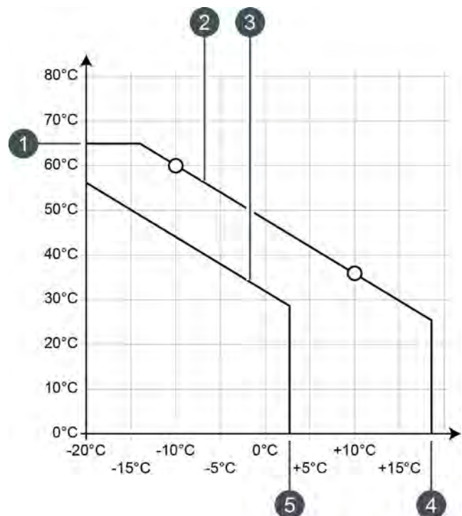
Fig. 8-17: Courbe de chauffage [Nuit]
