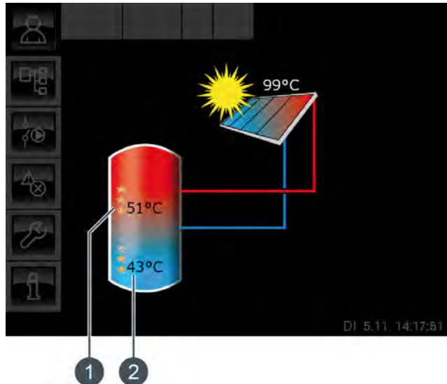
Fig. 8-25: Ballon tampon avec 2 serpents
