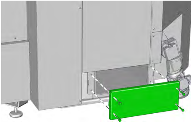
Fig. 7-2: Trappe de visite de la chambre d'inversion
