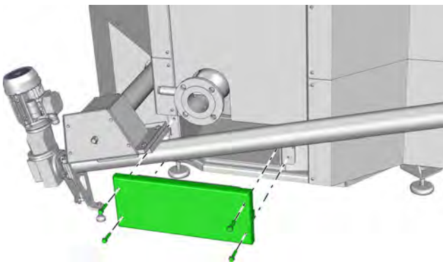
Fig. 7-3: Trappe de visite de la chambre d'inversion
