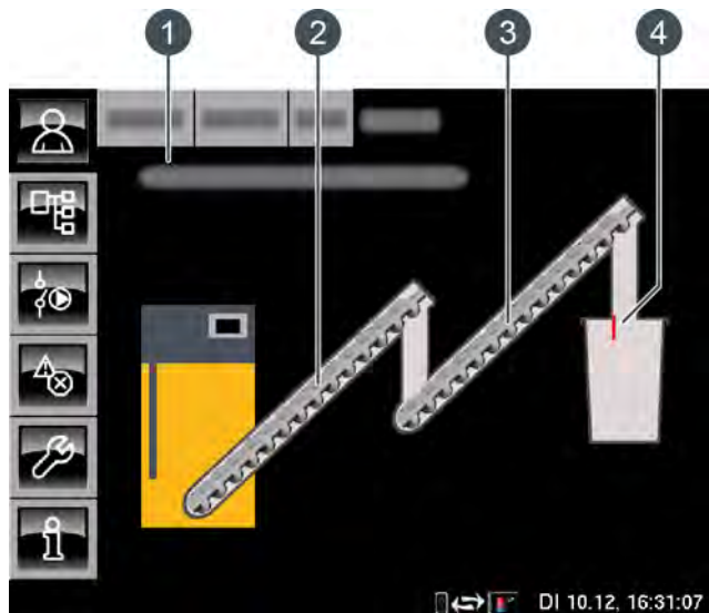
Fig. 8-37: Vue du décendrage externe
