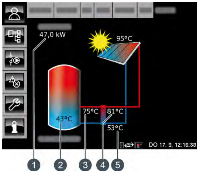
Fig. 8-26: Installation solaire avec échangeur thermique externe
