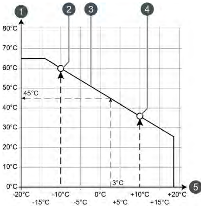
Fig. 8-16: Courbe de chauffage [Jour]
