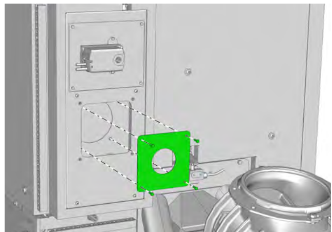
Fig. 7-6: Diaphragmes pour le recyclage des fumées, selon le combustible employé
