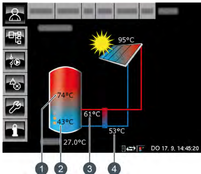
Fig. 8-27: Échangeur thermique externe avec vanne de stratification
